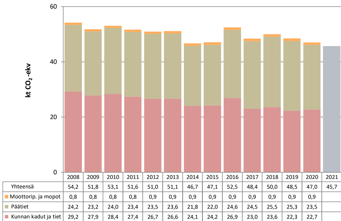
Kuva 8. Tieliikenteen päästöt Järvenpäässä vuosina 2008–2021. Vuoden 2021 tieto on ennakkotieto, joka perustuu liikennemäärien muutoksiin kunnan alueella.
