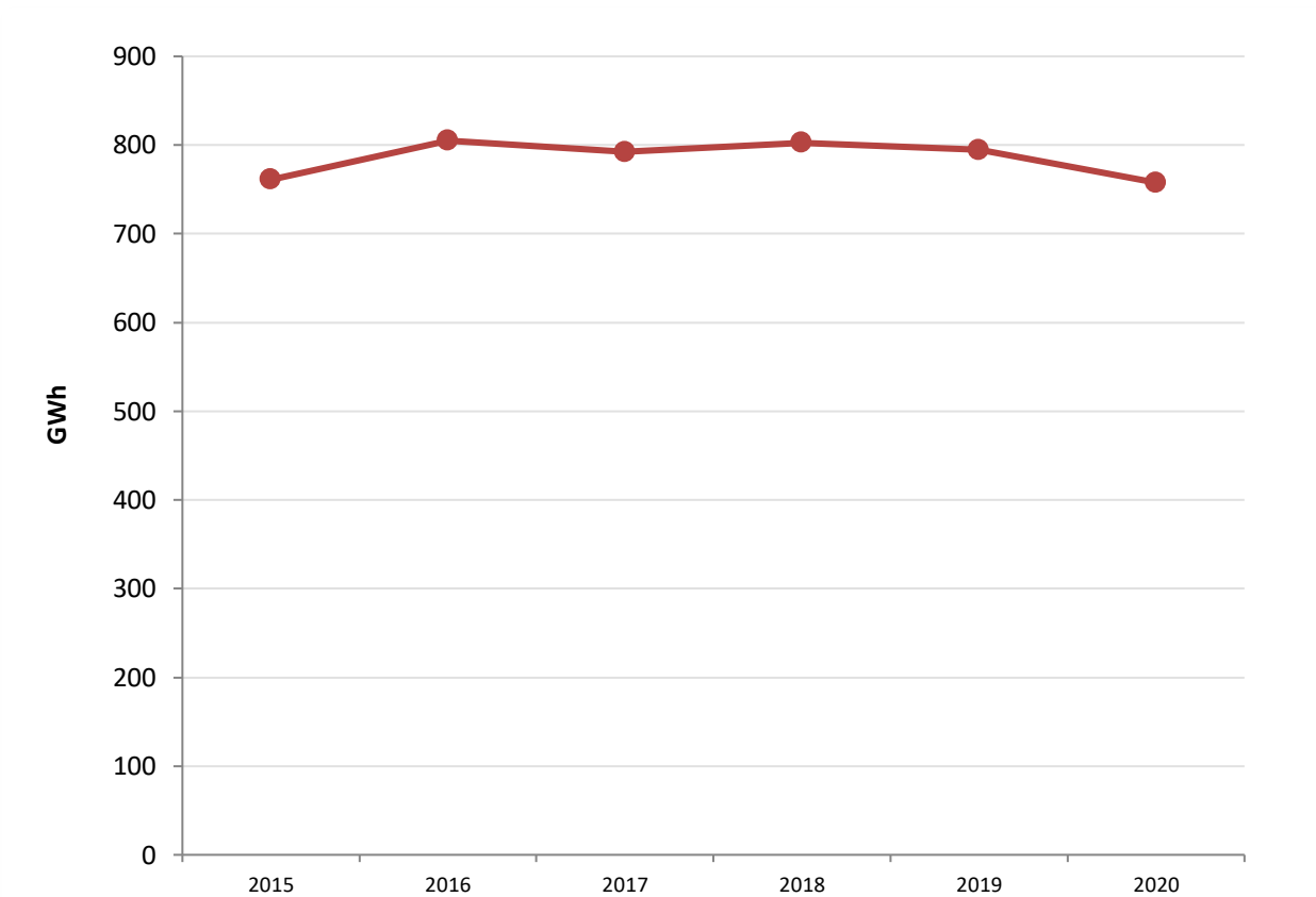
Kuva 24. Energian loppukulutuksen kehitys Järvenpäässä vuosina 2015–2020 ilman teollisuutta. Energian loppukulutus ei sisällä lämpöpumppujen tuottamaa uusiutuvaa energiaa, mutta sisältää niiden käyttämän sähkön.
