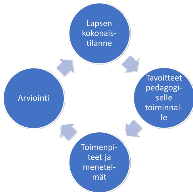
Kuva 4 Tuen arviointiprosessi
