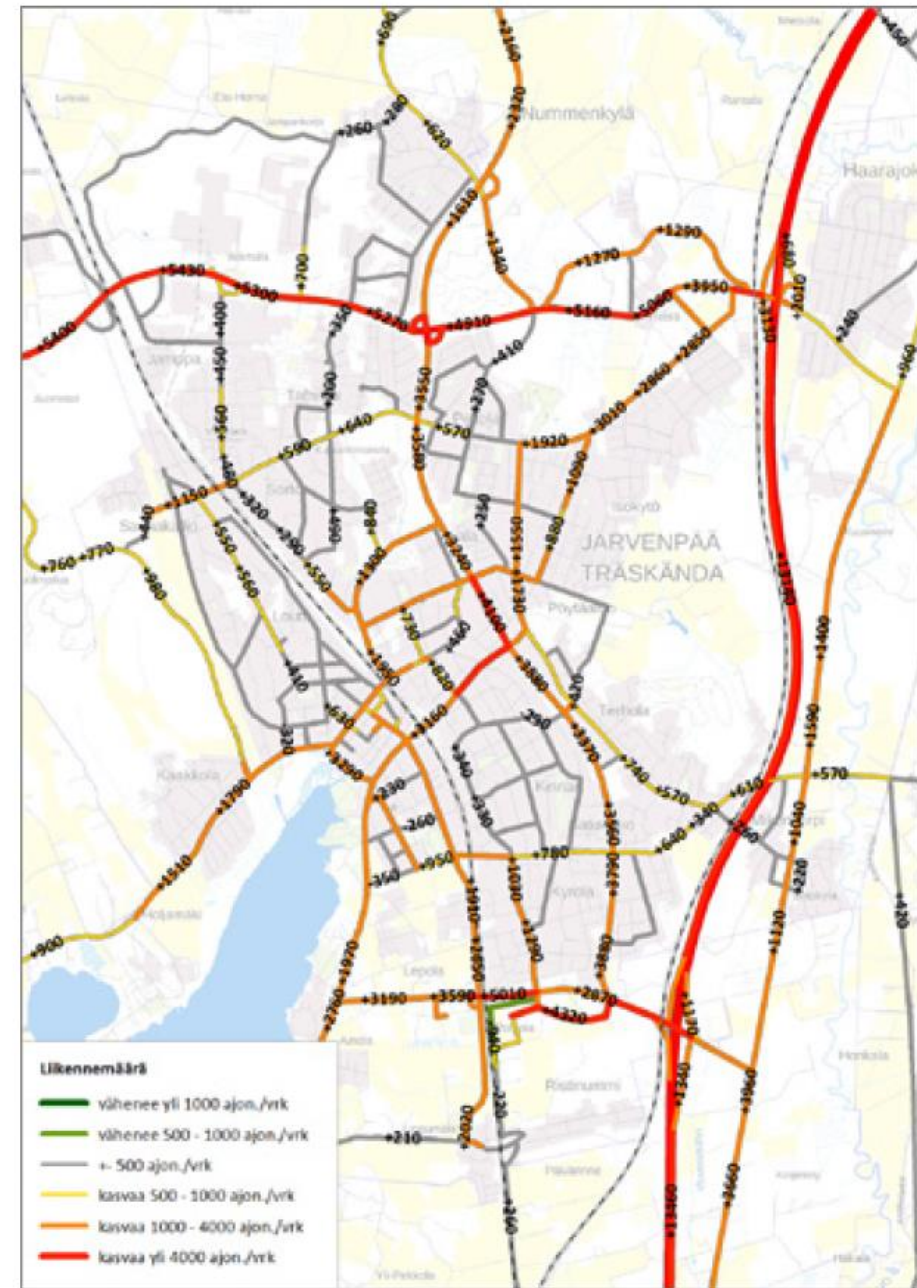
Kuva 20. Vuoden 2040 ennustettu liikennemäärä kaupungin katuverkolla ja liikennemäärien ennustettu kasvu nykytilasta vuoteen 2040 (Sitowise 2020a)
