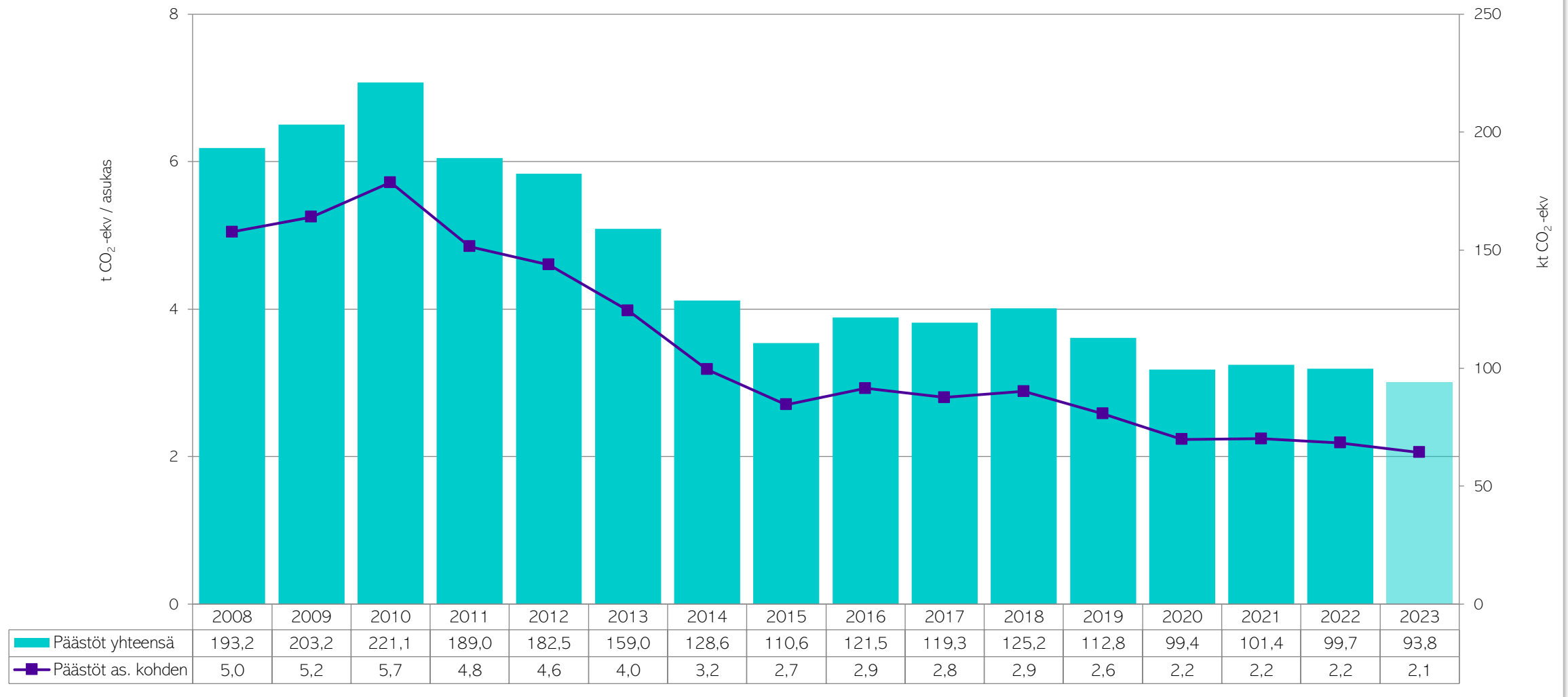
Kuva 3. Päästöt yhteensä ja asukasta kohden Järvenpäässä vuosina 2008–2023 ilman teollisuutta. Vuoden 2023 tieto on ennakkotieto. (CO 2 -raportti, 2024).
