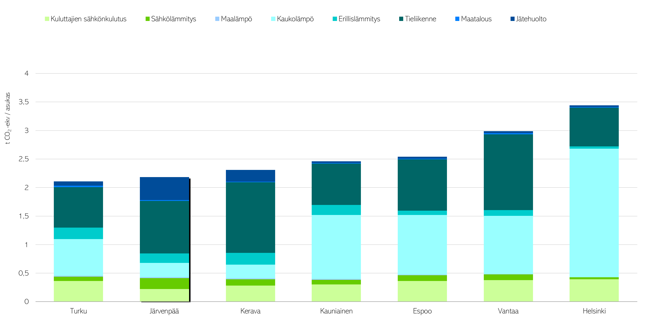
Kuva 11. Asukaskohtaisten päästöjen (t CO 2 -ekv/asukas) vertailu (ilman teollisuutta) vuonna 2022 sellaisissa CO 2 -raportin kunnissa, joissa on yli 500 asukasta maaneliökilometrillä. (CO 2 -raportti, 2024).
