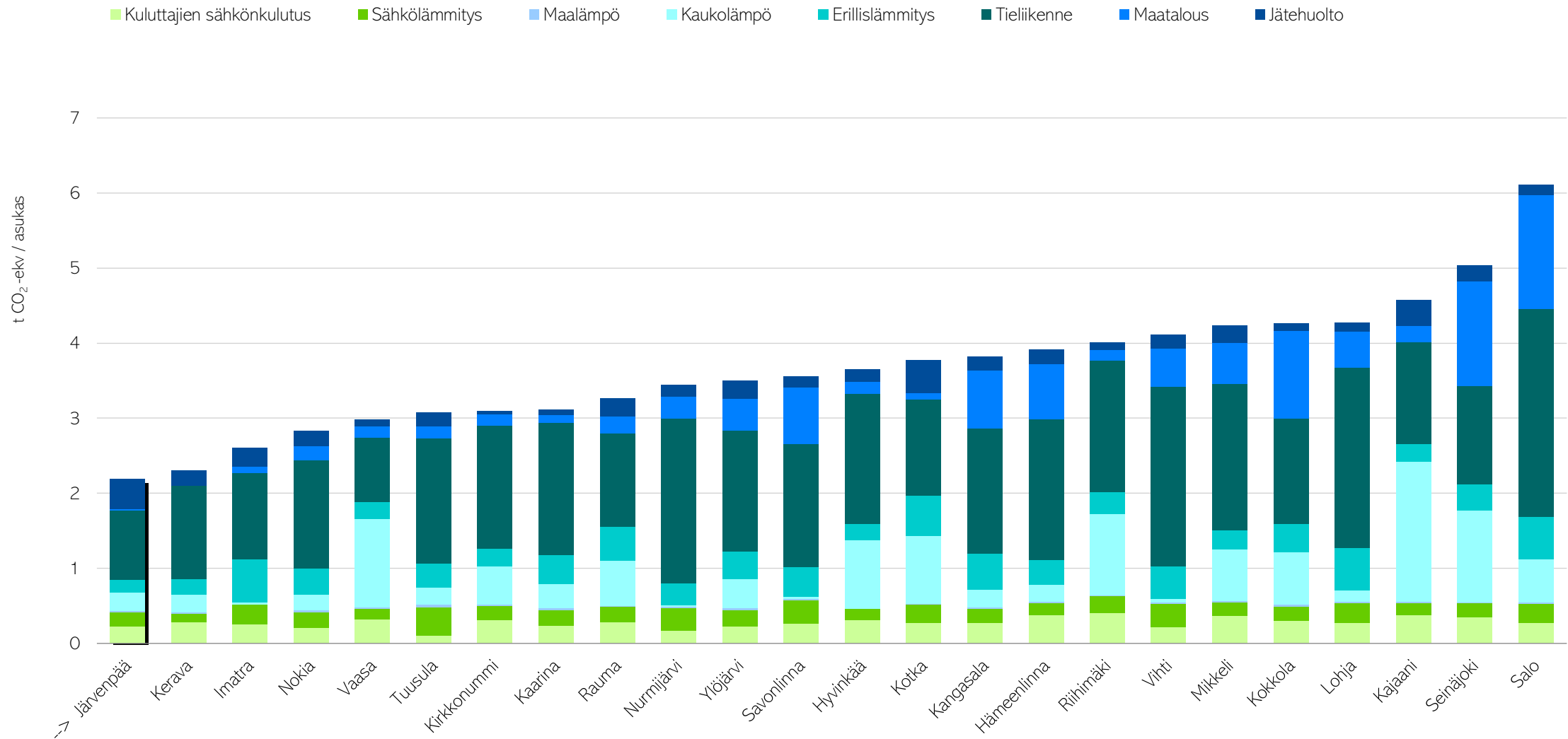
Kuva 10. CO2-raportissa mukana olevien 25 000–70 000 asukkaan kuntien asukaskohtaiset päästöt (t CO 2 -ekv/asukas) vuonna 2022 ilman teollisuutta. (CO 2 -raportti, 2024).
