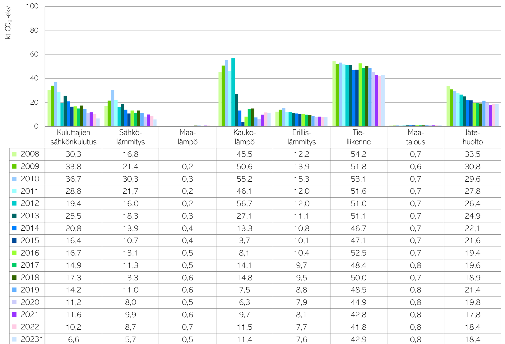
Kuva 2. Päästöt sektoreittain Järvenpäässä vuosina 2008–2023 ilman teollisuutta. Vuoden 2023 tieto on ennakkotieto. (CO 2 -raportti, 2024).
